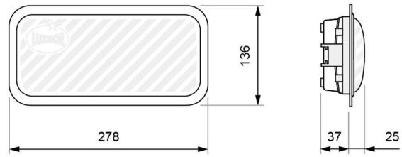
Montaje estanco
